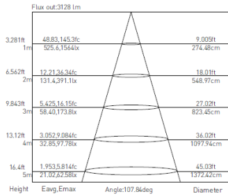
4-50W-X / 5-50W-X
