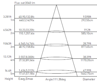
5-45W-X
